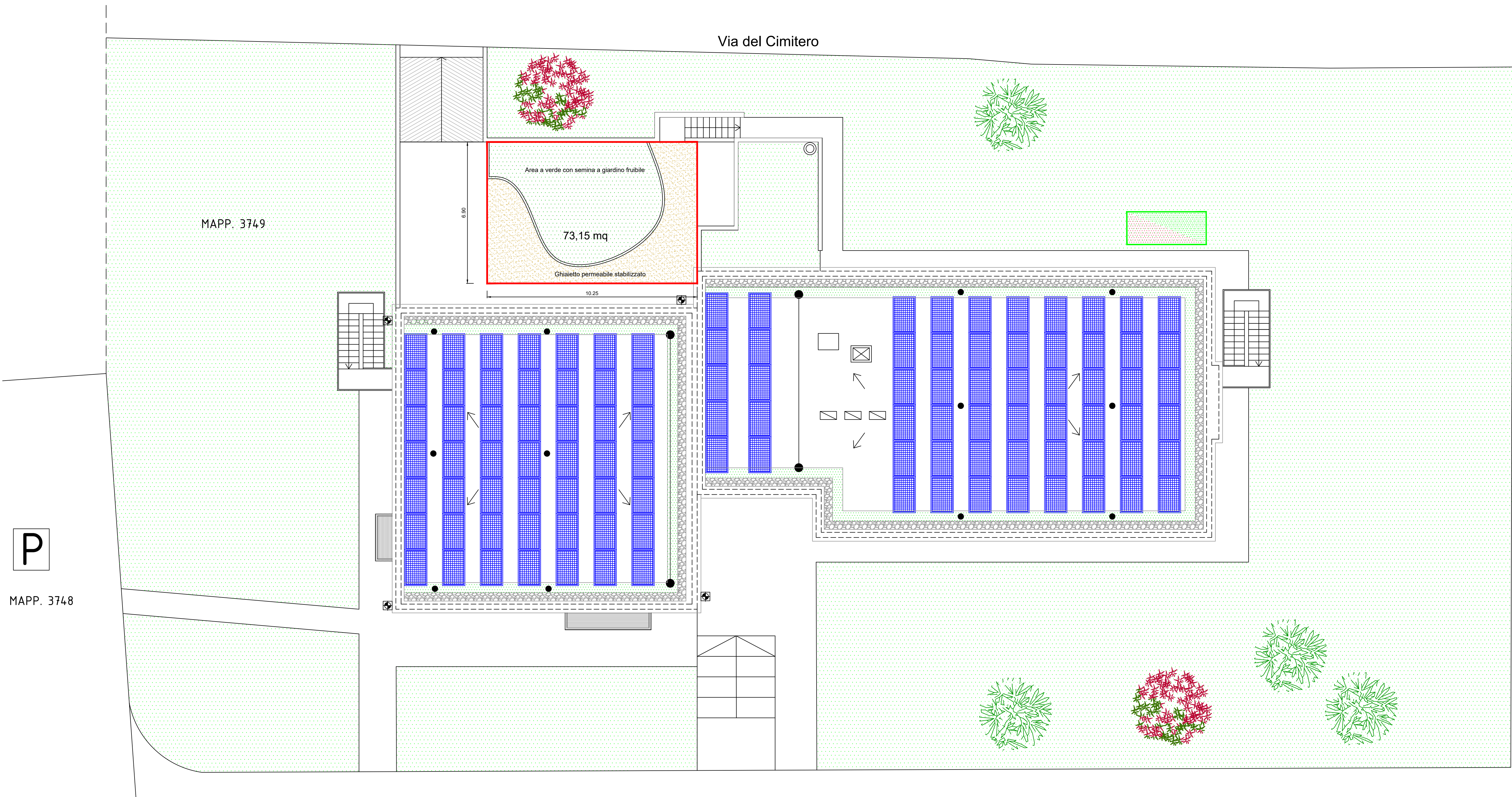
PLANIMETRIA GENERALE STATO DI PROGETTO
